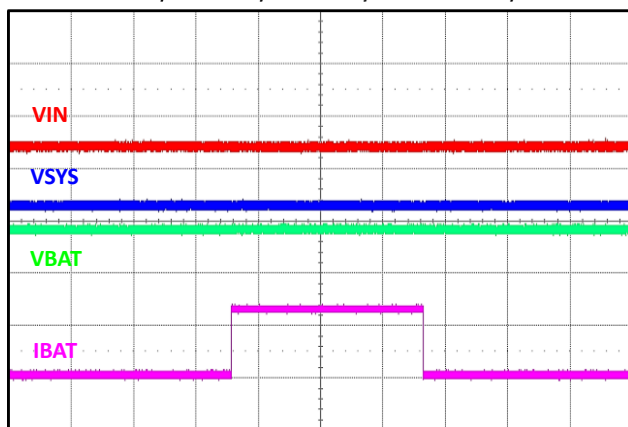
V_{BAT}=3.7V , I_{SYS}=0A Charge Enable/Disable
