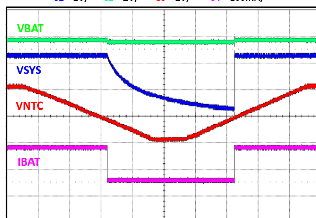
V_{BAT}=3.7V , I_{SYS}=0A PCB_OTP @Charge mode
