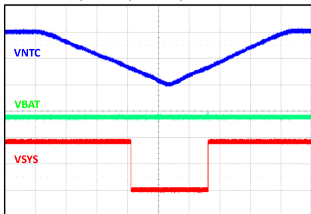
V_{IN}=0V , V_{BAT}=3.7V PCB_OTP @Discharge mode
