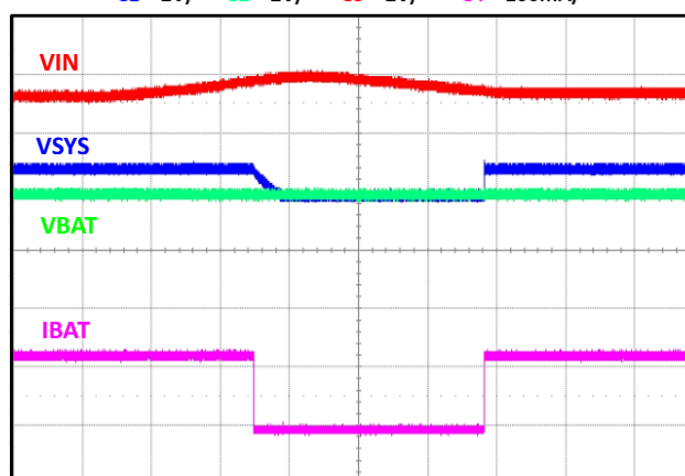
V_{BAT}=3.7V , I_{SYS}=0A V_{IN} OVP Operation
