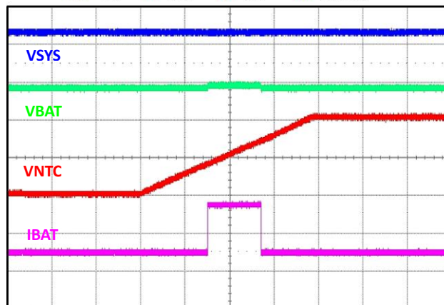
V_{BAT}=3.7V , I_{SYS}=0A , PCB_OTP disabled NTC Rising
