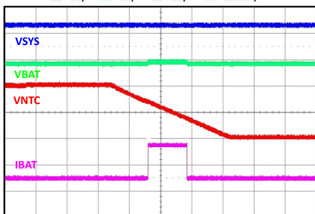
V_{BAT}=3.7V , I_{SYS}=0A , PCB_OTP disabled NTC Falling
