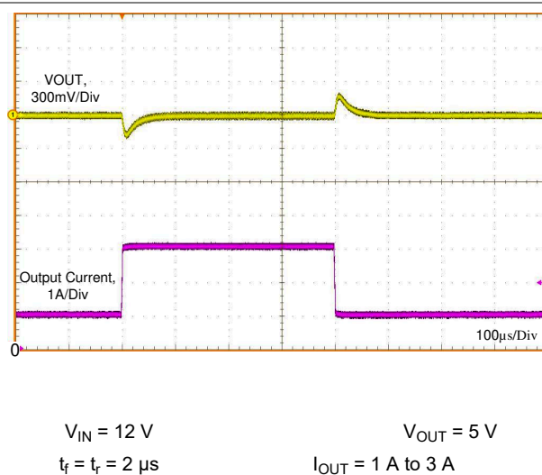
图 8-16. Load Transient
