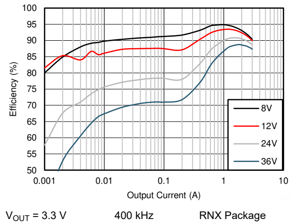
图 8-6. Efficiency
