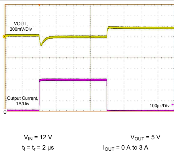
图 8-15. Load Transient
