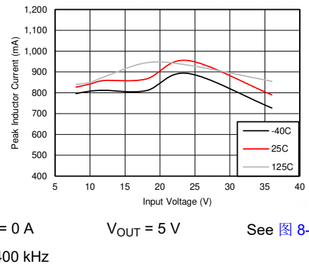
图 6-6. I_{PEAK-MIN}
