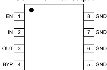
SOIC-8
