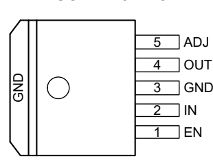
TO-263-5B
