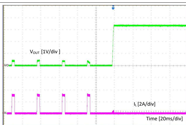
图 21. Short Recovery
