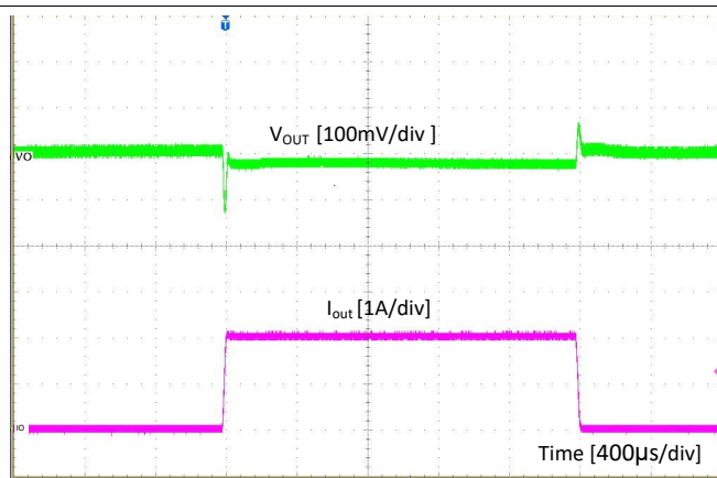
图 19. Load Transient
