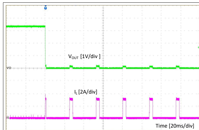
图 20. Short Protection
