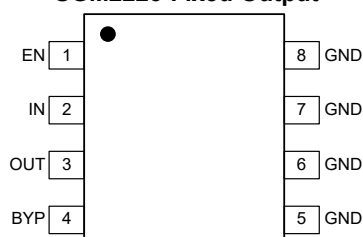
SOIC-8
