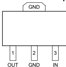
SOT-89-3
