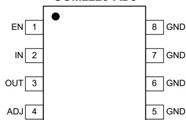
SOIC-8
