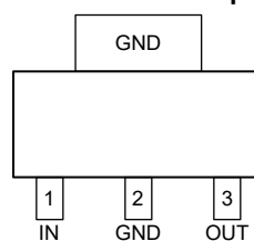
SOT-223-3
