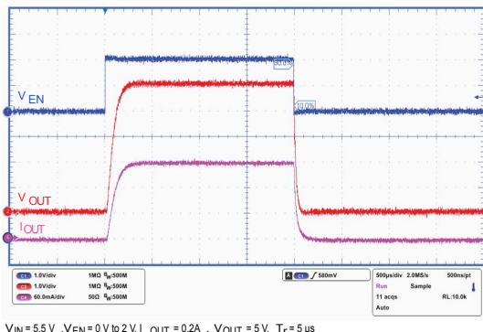
Figure 20. Enable startup ( V_{OUT} = 5\text{ V} )
