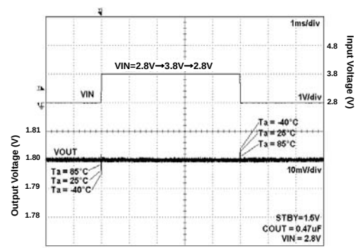
Fig 77. VIN Response
