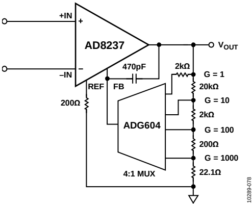
图76. 采用多路复用器的可编程增益
