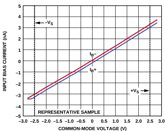
图15. 输入偏置电流与共模电压的关系
