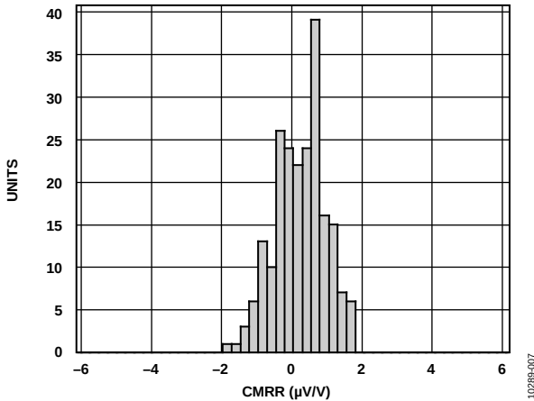
图7. CMRR的典型分布图
