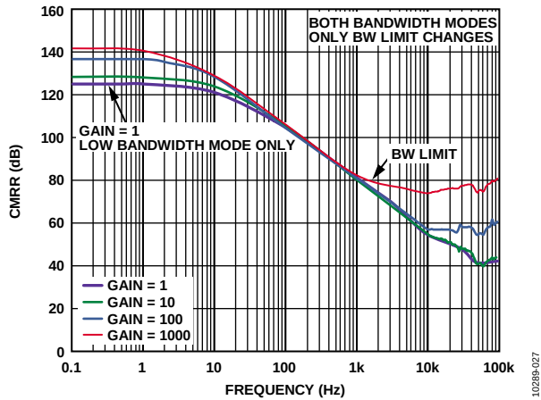
图28. CMRR与频率的关系
