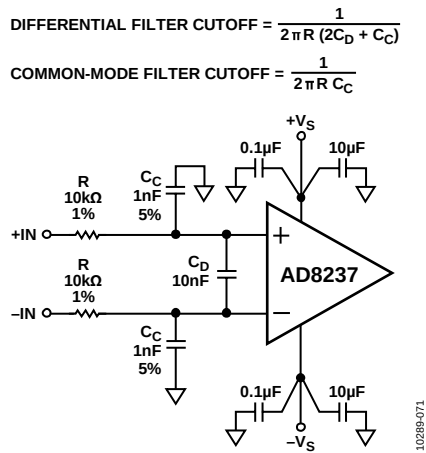
图69. 添加额外的RFI滤波功能
