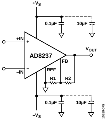
图73. 电源去耦、REF及输出以局部地为参考
