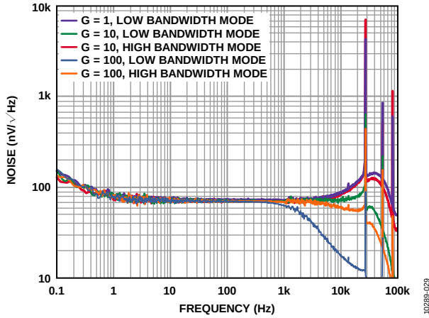
图30. 电压噪声谱密度与频率的关系
