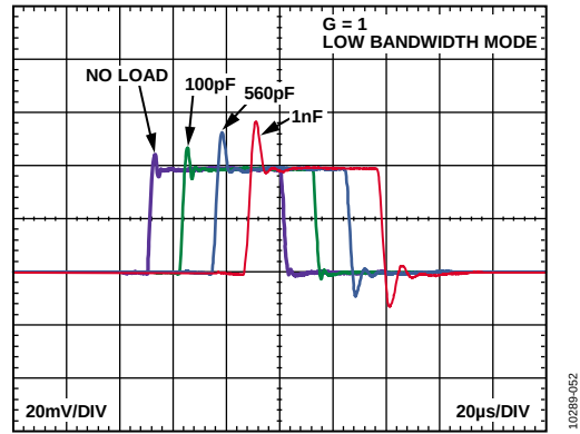
图50. 各种容性负载条件下的小信号脉冲响应, G = 1 , R_L = \infty , 低带宽模式
