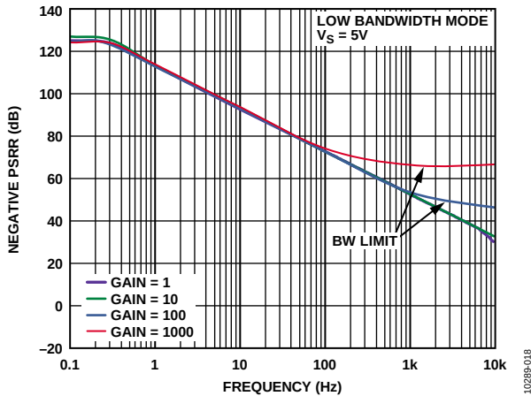
图18. 负PSRR与频率的关系, RTI, 低带宽模式, V_S = 5V
