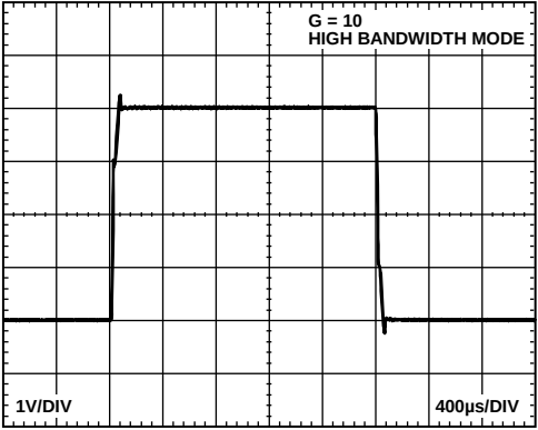
图43. 大信号脉冲响应，高带宽模式， G = 10 , R_L = 10\text{ k}\Omega , C_L = 10\text{ pF}
