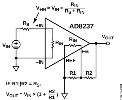
图67. 消除输入阻抗误差
