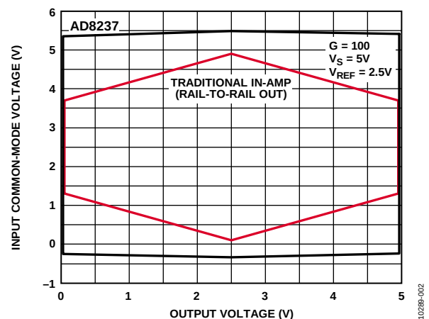
图2. 输入共模电压与输出电压的关系(+ V_S = 5\text{ V} , G = 100 )
