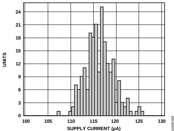
图9. 电源电流的典型分布图
