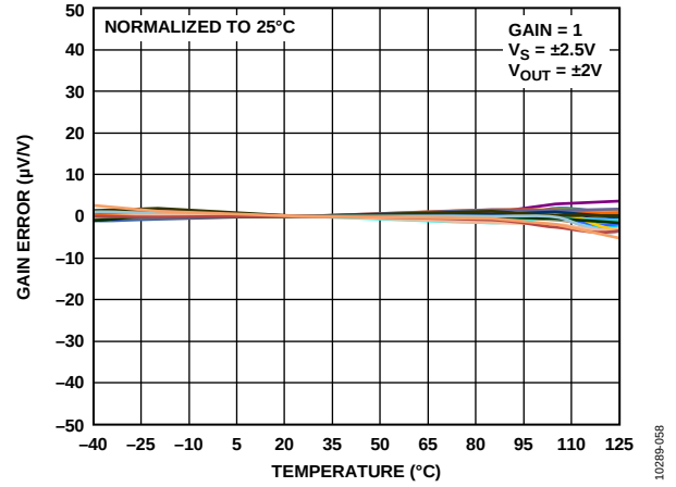
图56. 增益与温度的关系
