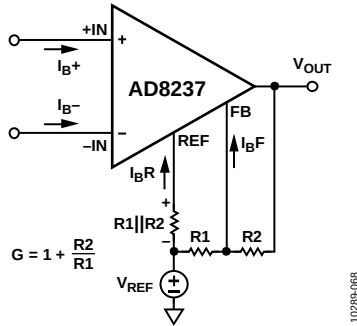
图66. 消除FB输入偏置电流的误差
