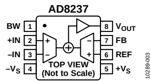
图3. 引脚配置
