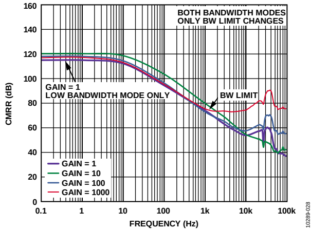
图29. CMRR与频率的关系, 1 kΩ非均衡信号源
