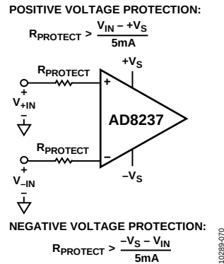
图68. 针对大输入电压的保护电阻
