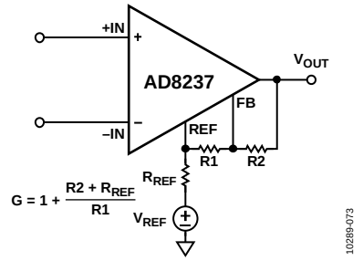
图71. 使用基准电阻计算增益
