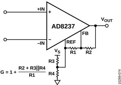
图72. 使用分压器设置基准电压
