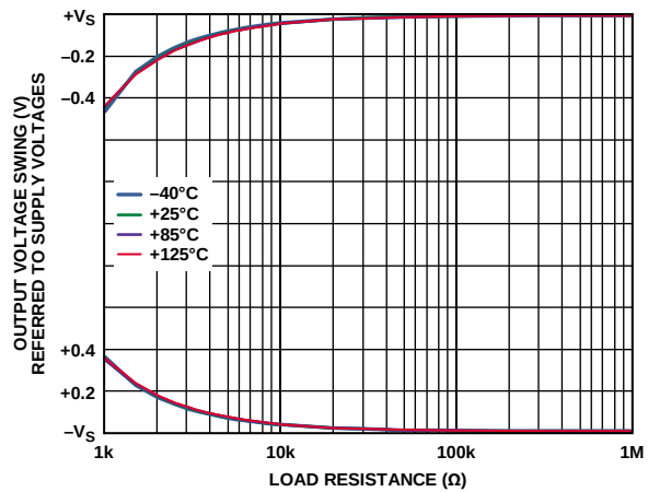
图61. 输出电压摆幅与负载阻抗的关系, V_s = \pm 2.5\text{ V}
