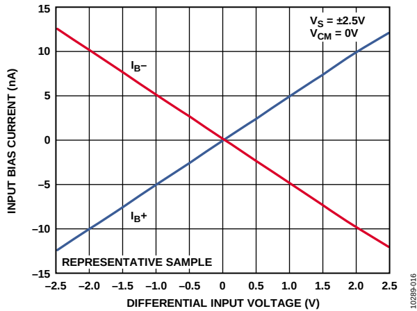
图16. 输入偏置电流与差分输入电压的关系
