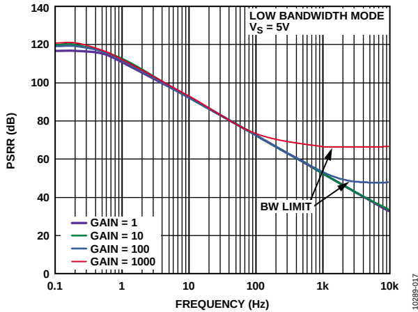
图17. 正PSRR与频率的关系, RTI, 低带宽模式, V_S = 5V
