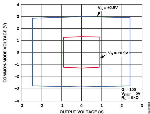
图13. 输入共模电压与输出电压的关系, G=100 , V_{REF}=0V , V_S=\pm 2.5V 和 V_S=\pm 0.9V , R_L=5k\Omega 至地
