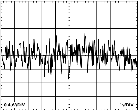
图31. 0.1 Hz至10 Hz折合到输入端电压噪声
