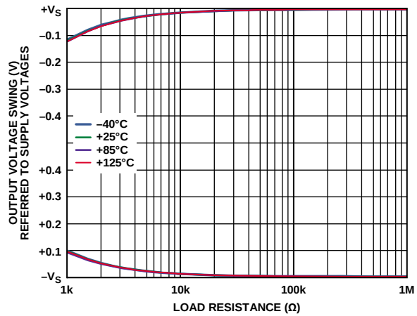
图62. 输出电压摆幅与负载阻抗的关系, V_s = \pm 0.9\text{ V}
