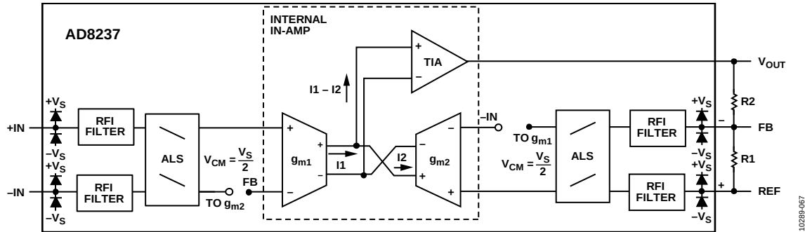
图65. 原理示意图
