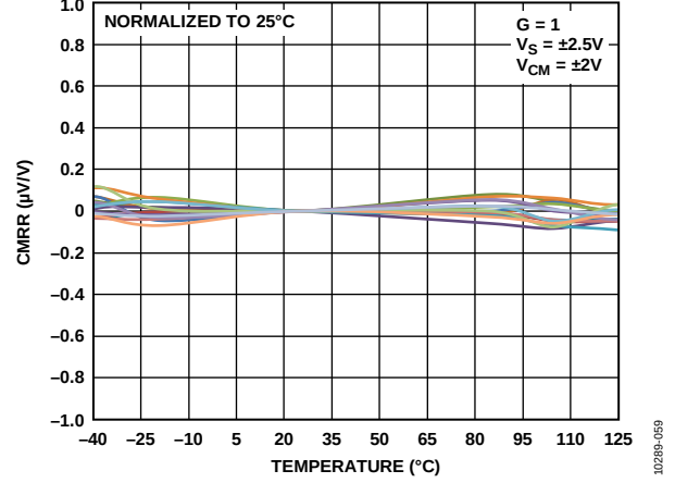
图57. CMRR与温度的关系
