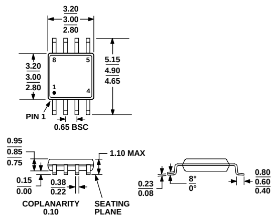
COMPLIANT TO JEDEC STANDARDS MO-187-AA 图78. 8引脚超小型封装[MSOP](RM-8) 尺寸单位：mm
