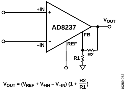
图70. 施加增益至基准电压
