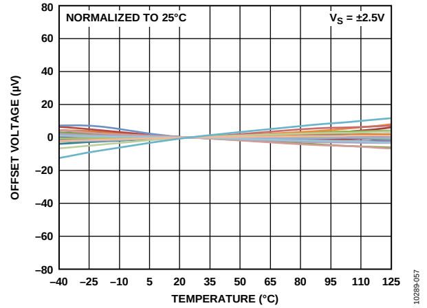
图55. 失调电压与温度的关系
