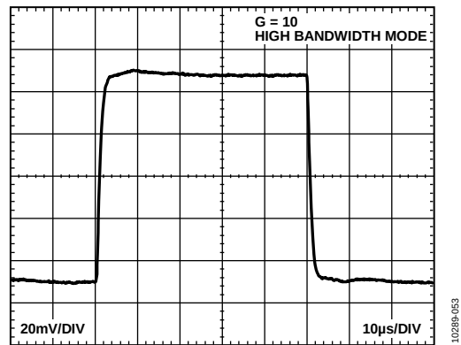
图51. 小信号脉冲响应, G = 10 , R_L = 10\text{ k}\Omega , C_L = 100\text{ pF} , 高带宽模式
