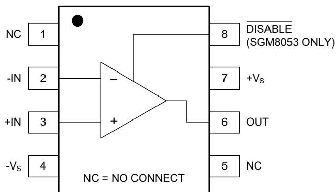
SOIC-8
