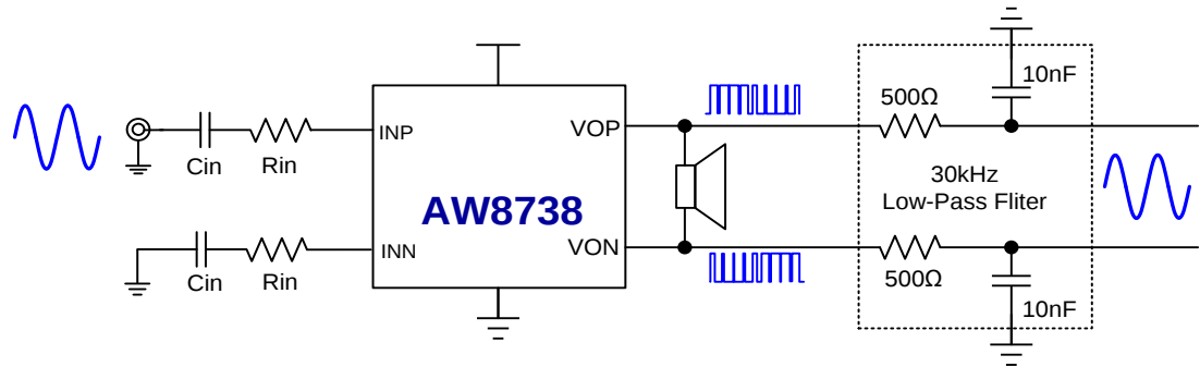
图 6 AW8738 测试电路图
