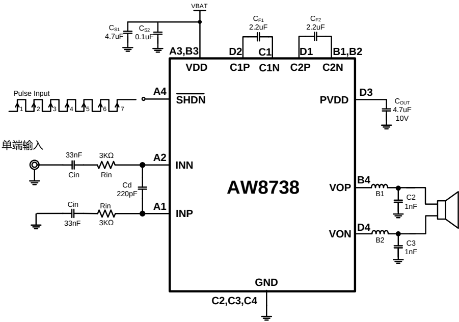
图 4 AW8738 单端输入方式应用图 (注1)
