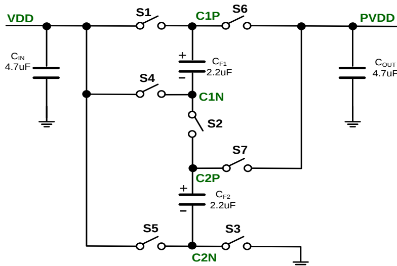
图 11 电荷泵原理图
