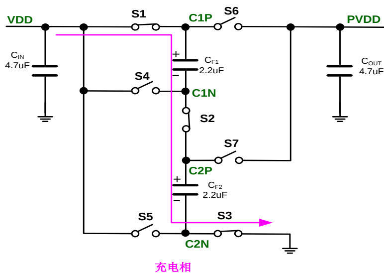
图 12 Φ1: Flying 电容充电
