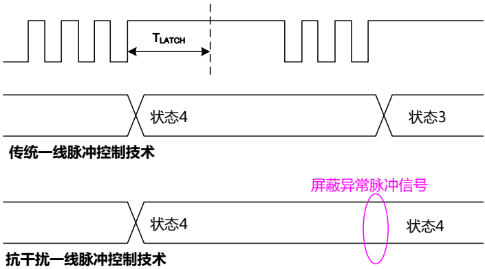
图 15 抗干扰一线脉冲功能示意图
