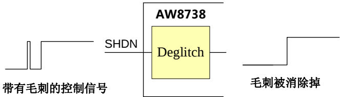
图 14 艾为 Deglitch 功能示意图
