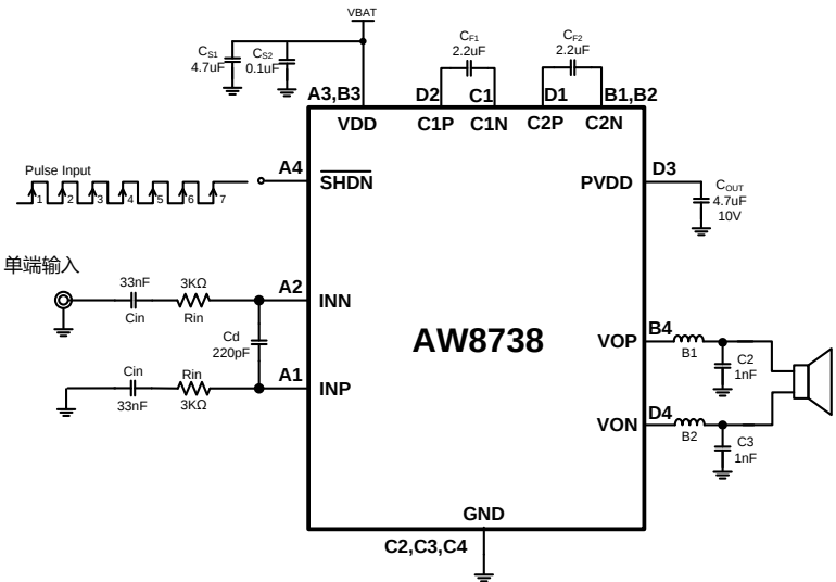
图 1 AW8738 单端输入方式应用图
