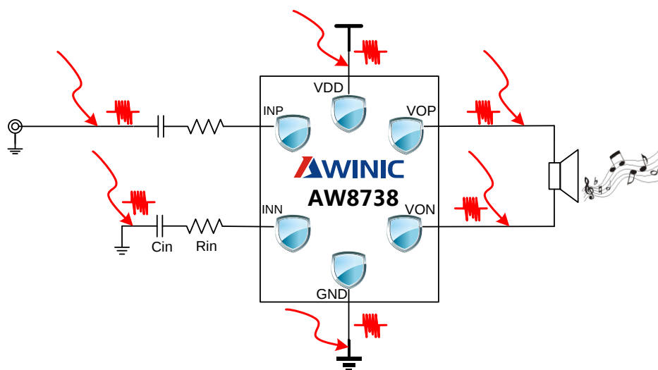
图 19 RF 辐射耦合示意图
