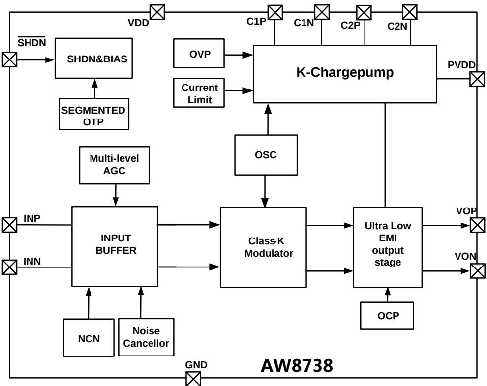
图 3 AW8738 功能框图
