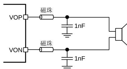
图 20 典型的输出磁珠、电容应用图
