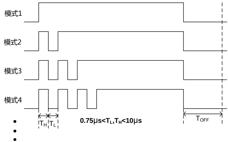
图 16 一线脉冲控制方法
