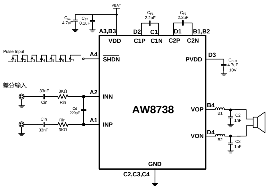
图 5 AW8738 差分输入方式应用图
