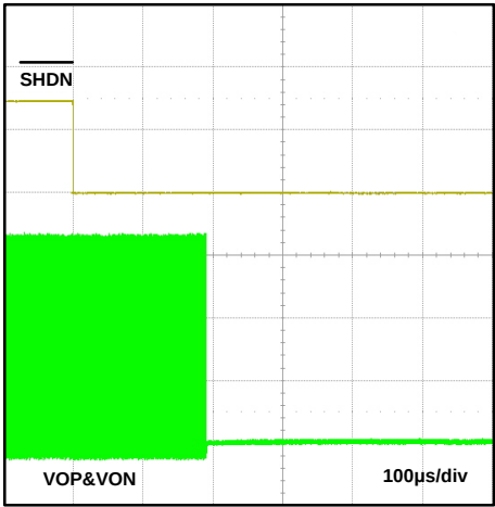
关断时序
