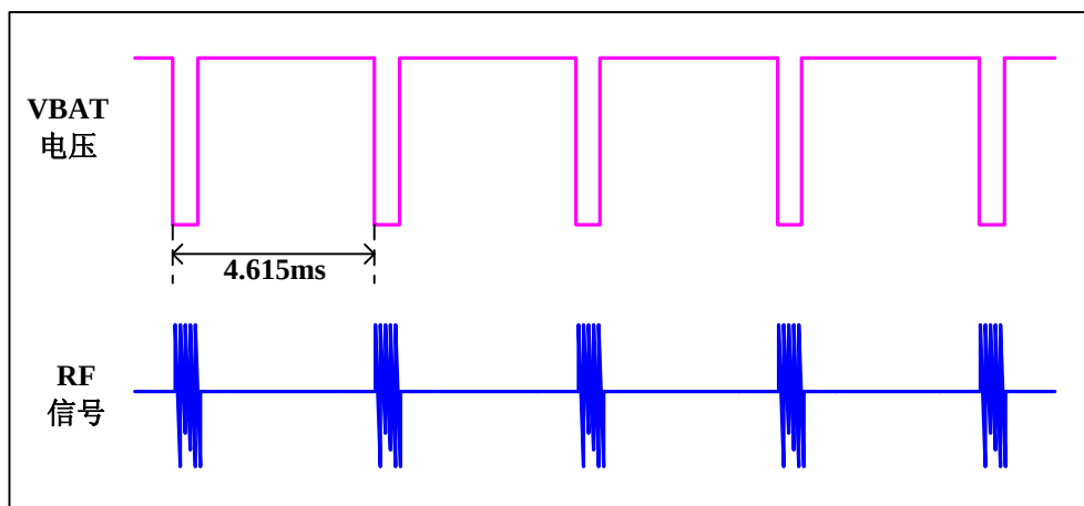
图 18 GSM 射频工作时电源电压和 RF 信号示意图
