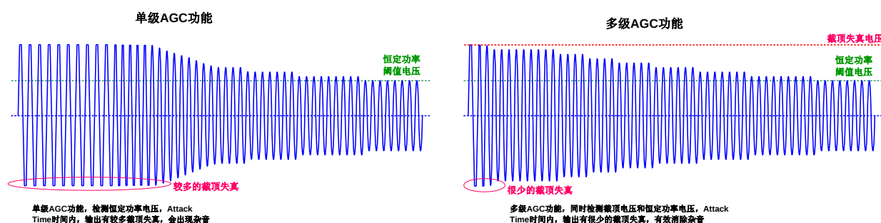
图 10 单级 AGC/多级 AGC 工作原理图
