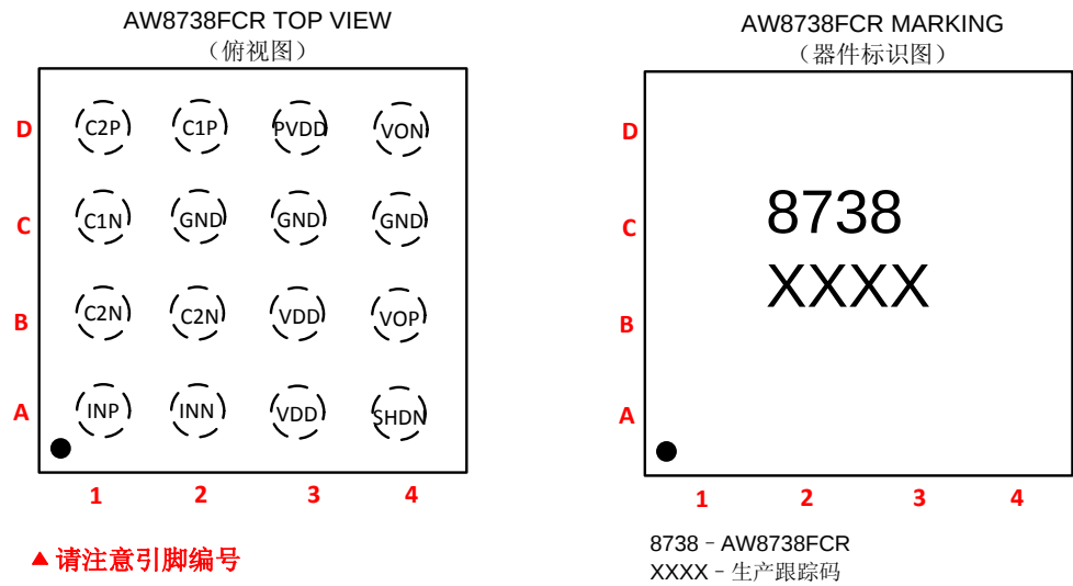
图 2 AW8738FCR 引脚分布俯视图及器件标识图
