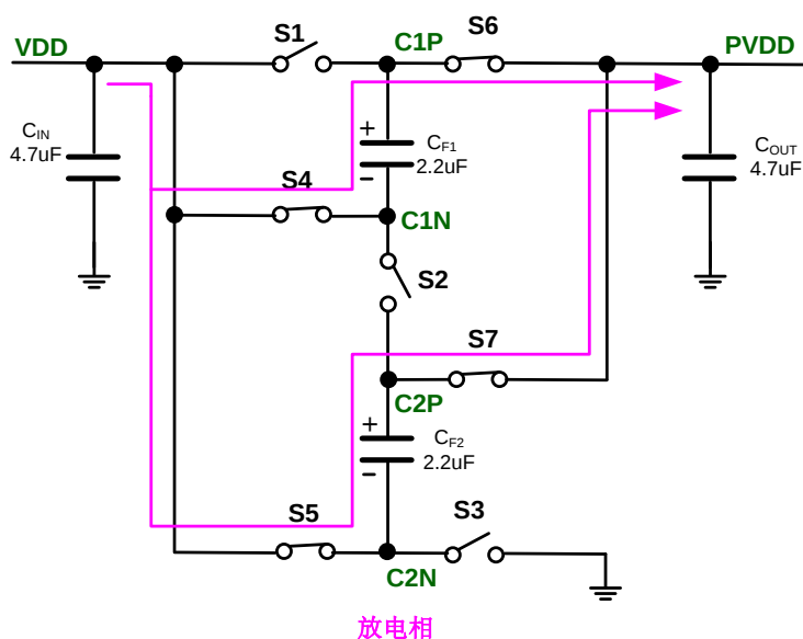
图 13 Φ2: Flying 电容电荷转移到输出电容 COUT
