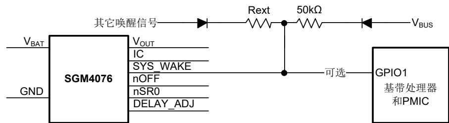
图5. 接入外部唤醒的连接方式之一
