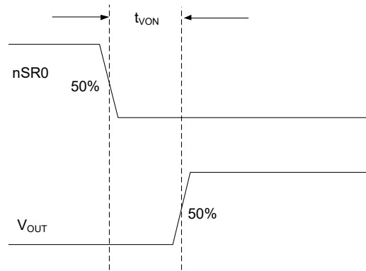
图 8. Turn-On with nSR0
