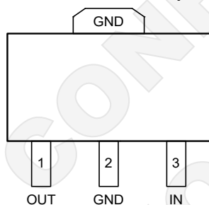
SOT-89-3
