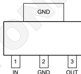
SOT-223-3
