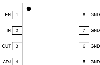
SGM2205-ADJ
