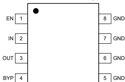
SGM2205-Fixed Output
